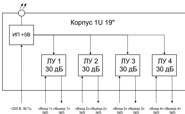
Рисунок – Функциональная схема изделия.
